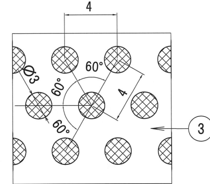
スクリーン詳細図(40メッシュ)
