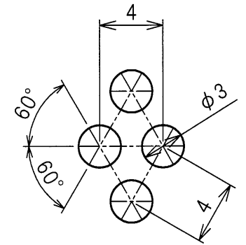
スクリーン詳細図
