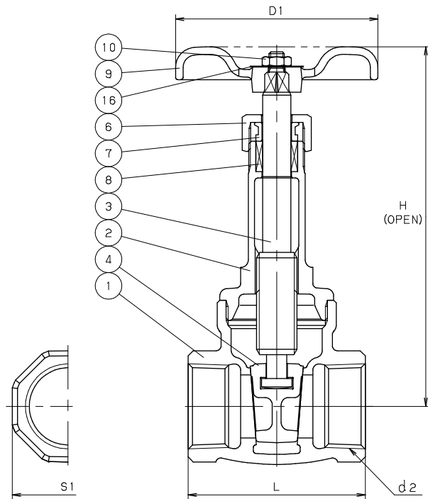
寸法表
