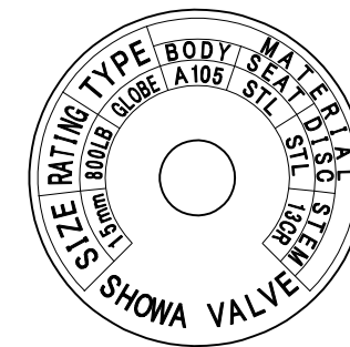
銘板表示例
