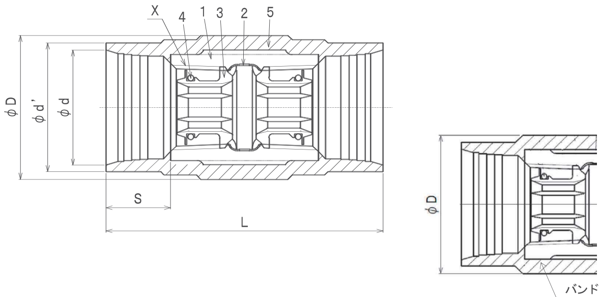
付図1. バンド有り製品の端部形状
