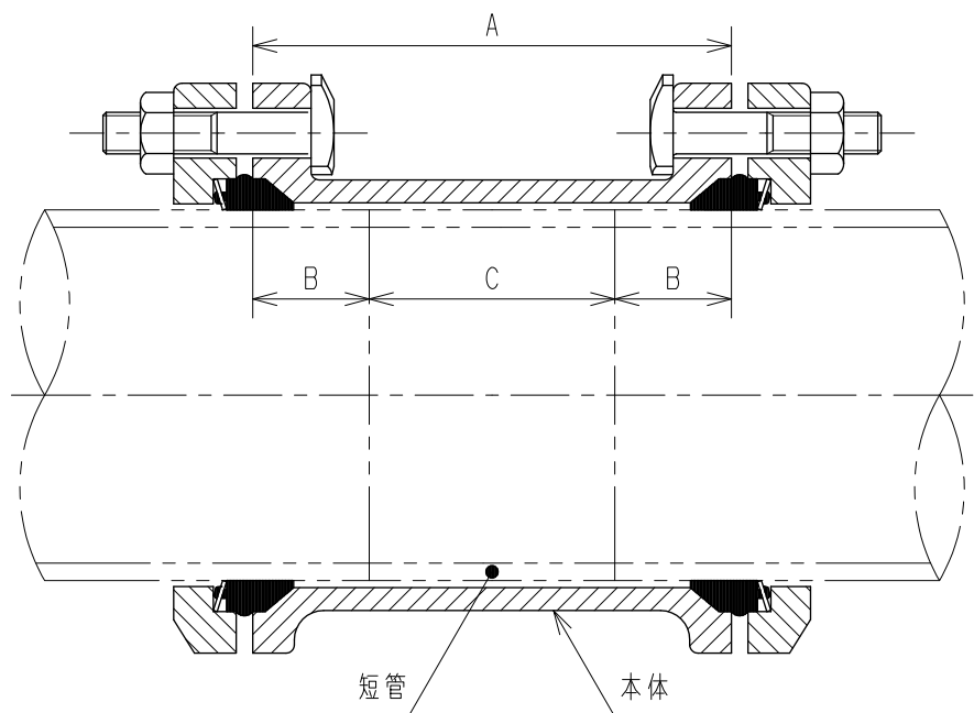
組立図
