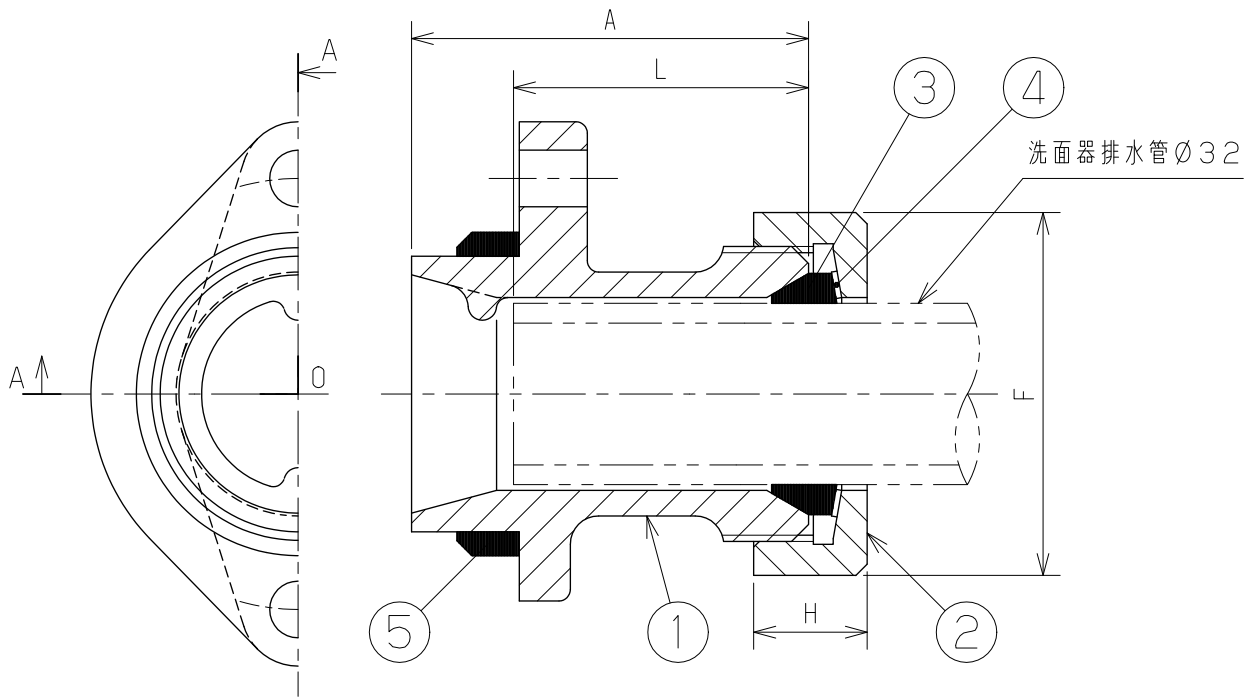
断面 A-0-A
