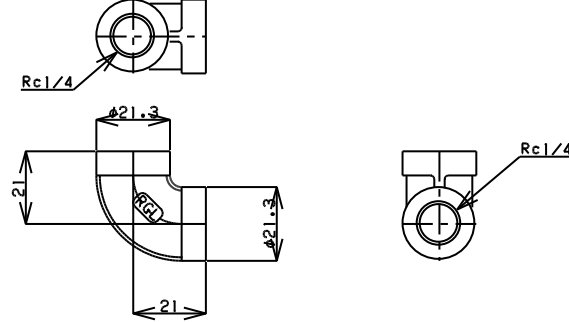
TITLE 90° エルボ MODEL R-1-1/4
