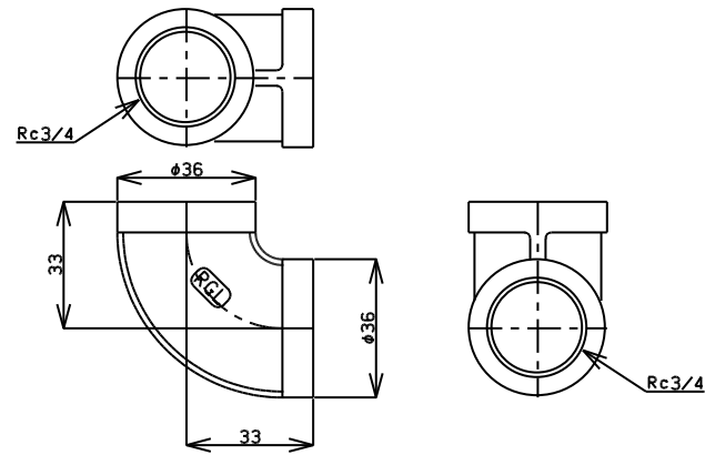
TITLE 90° エルボ MODEL R-1-3/4
