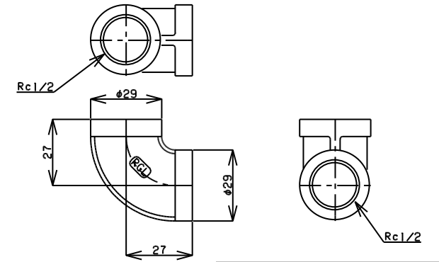
TITLE 90° エルボ MODEL R-1-1/2
