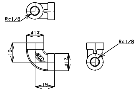
TITLE 90° エルボ MODEL R-1-1/8
