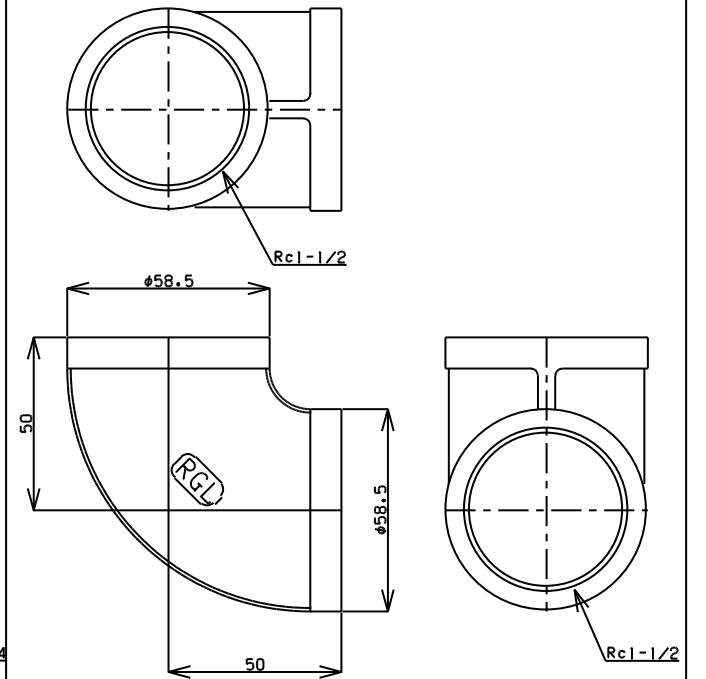
TITLE 90° エルボ MODEL R-1-1-1/2
