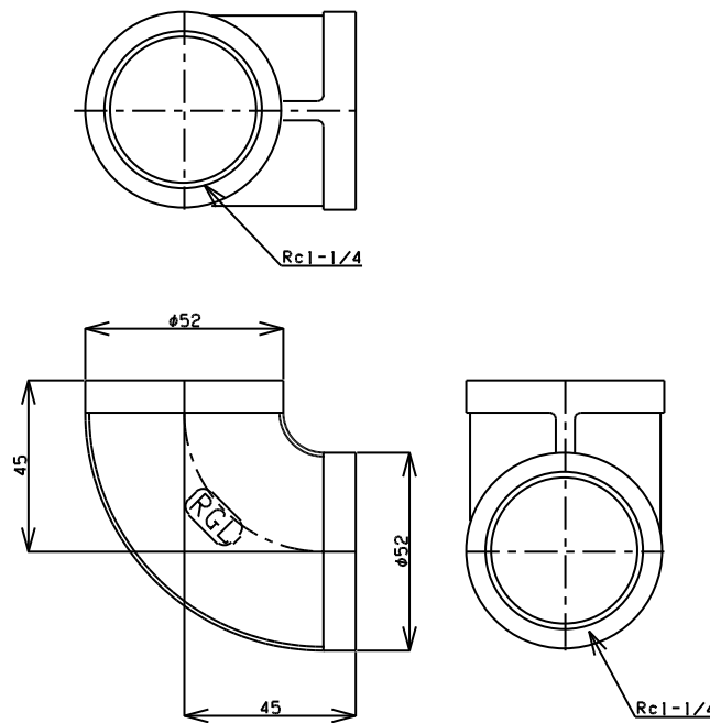
TITLE 90° エルボ MODEL R-1-1-1/4
