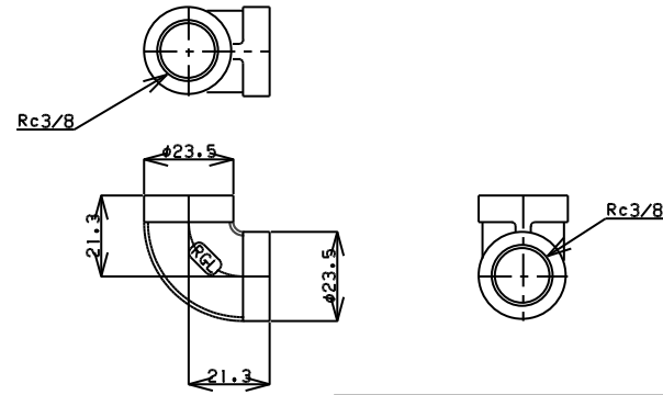
TITLE 90° エルボ MODEL R-1-3/8
