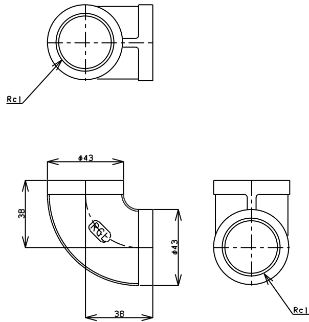
TITLE 90° エルボ MODEL R-1-1
