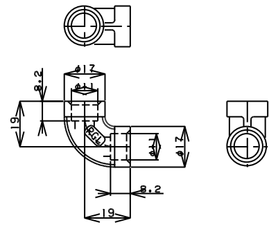
TITLE 溶接用90°エルボ MODEL R-1B-1/8
