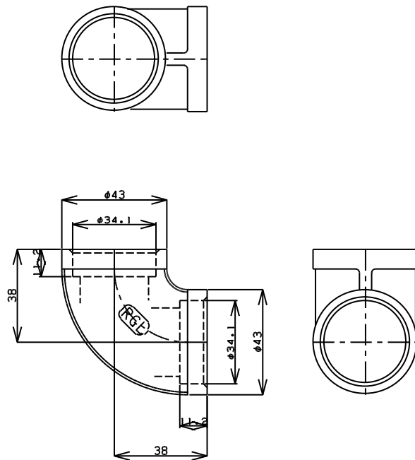
TITLE 溶接用90°エルボ MODEL R-1B-1
