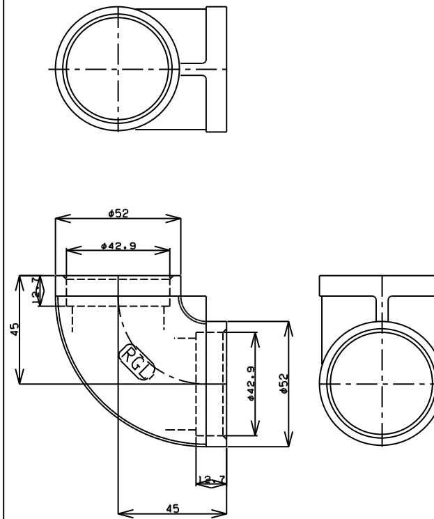
TITLE 溶接用90°エルボ MODEL R-1B-1-1/4
