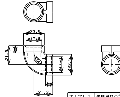
TITLE 溶接用90°エルボ MODEL R-1B-3/8
