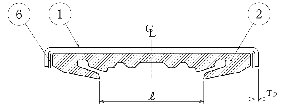
断面詳細図
