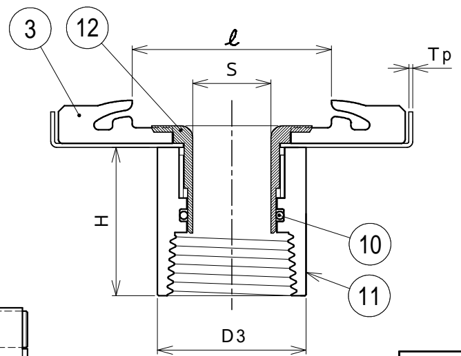
断面詳細図
