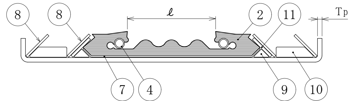
断面詳細図
