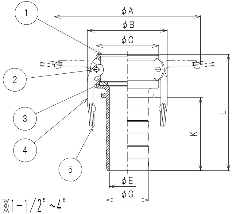
633-CT SST サイズ別寸法表 (単位: mm)
