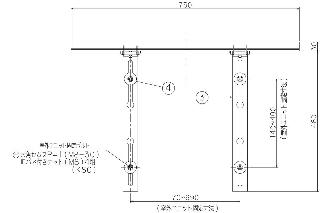
A 矢視図
