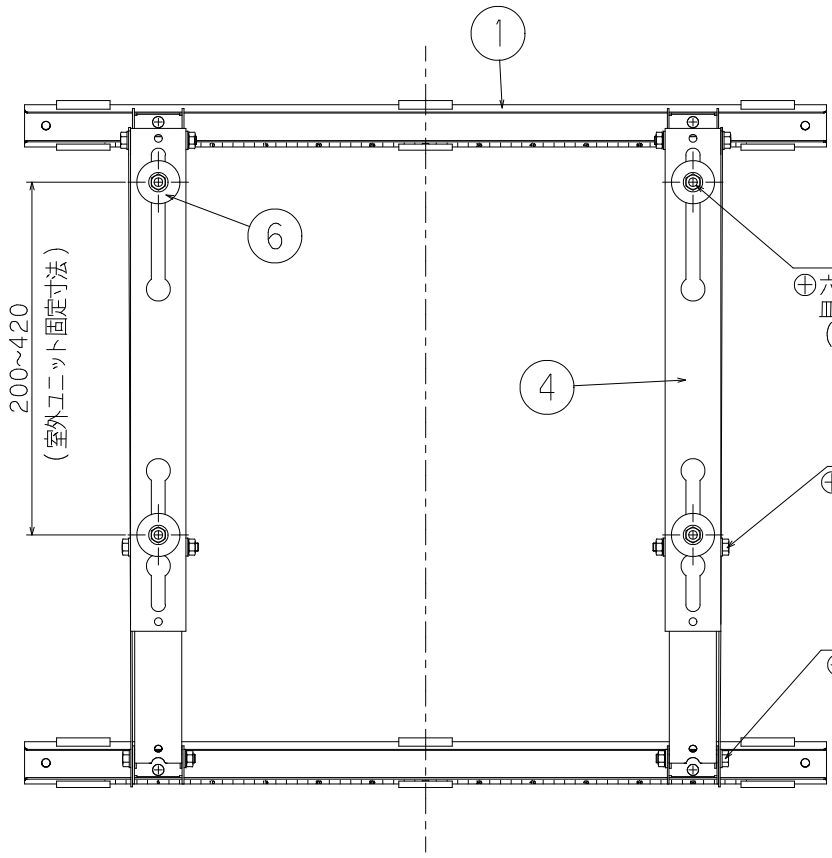
A 矢視図
