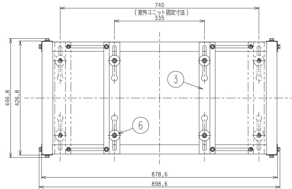
A 矢視図
