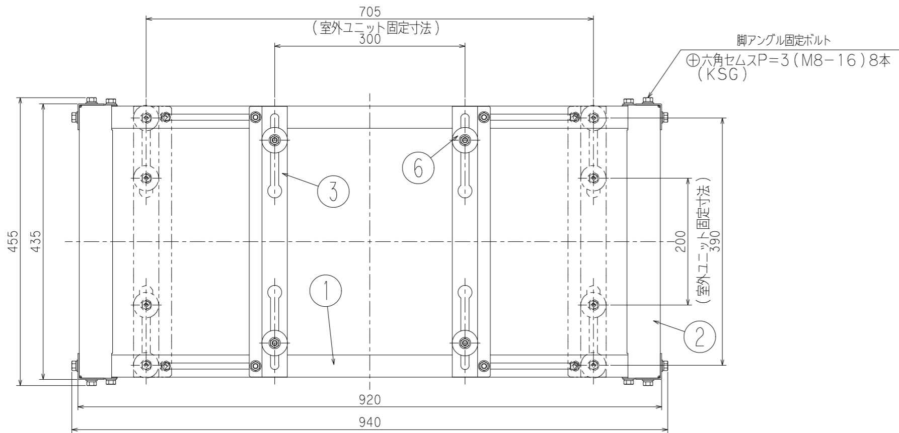
A 矢視図
