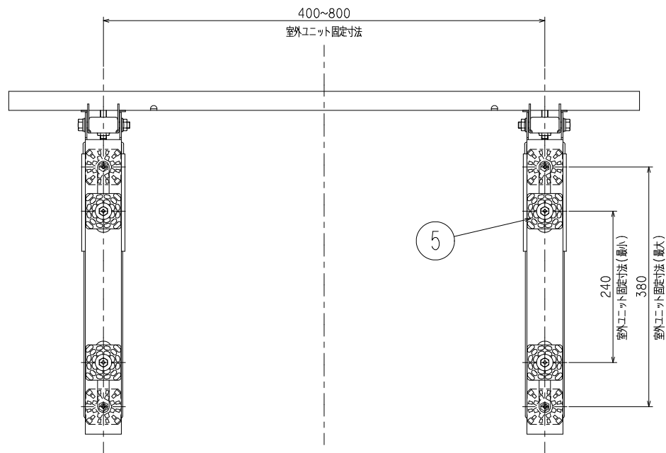
A 矢視図
