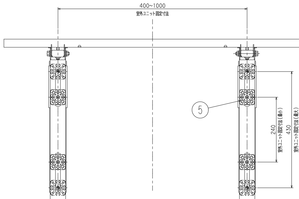
A 矢視図
