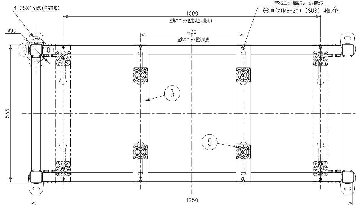
A 矢視図
