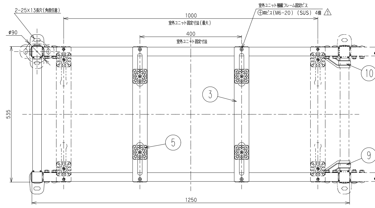
A 矢視図
