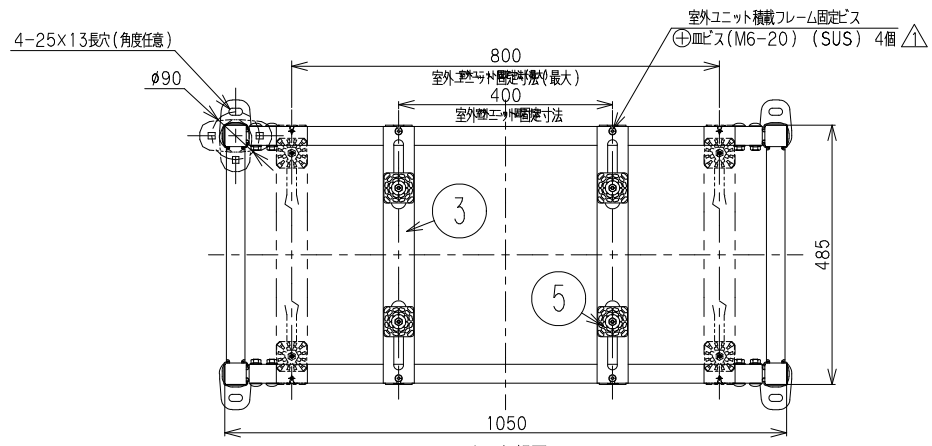
A 矢視図
