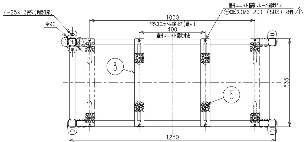
A 矢視図
