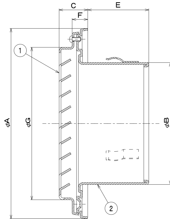
断面 A-A
