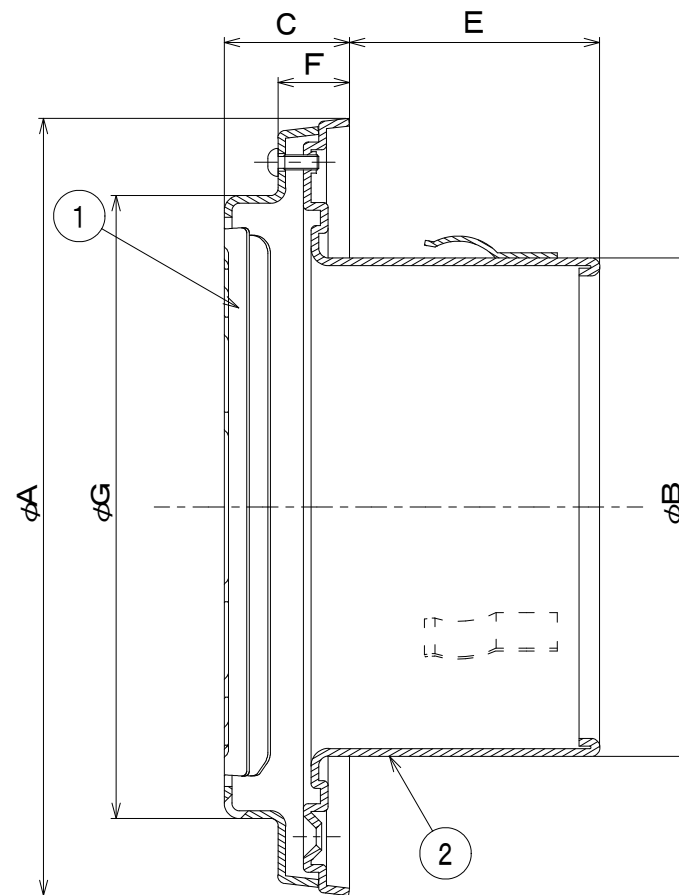
断面 A-A
