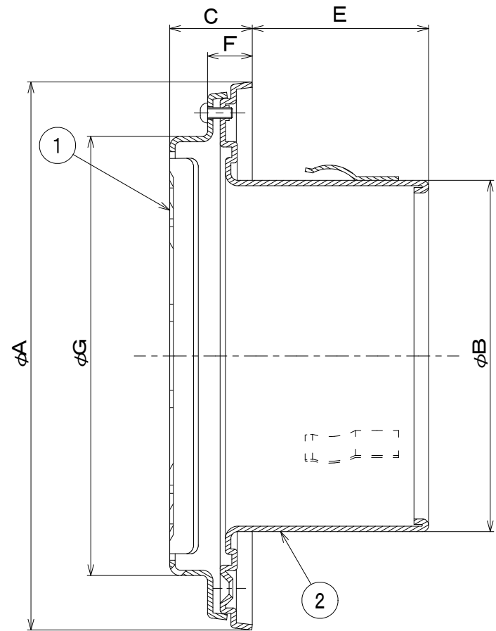
断面 A-A
