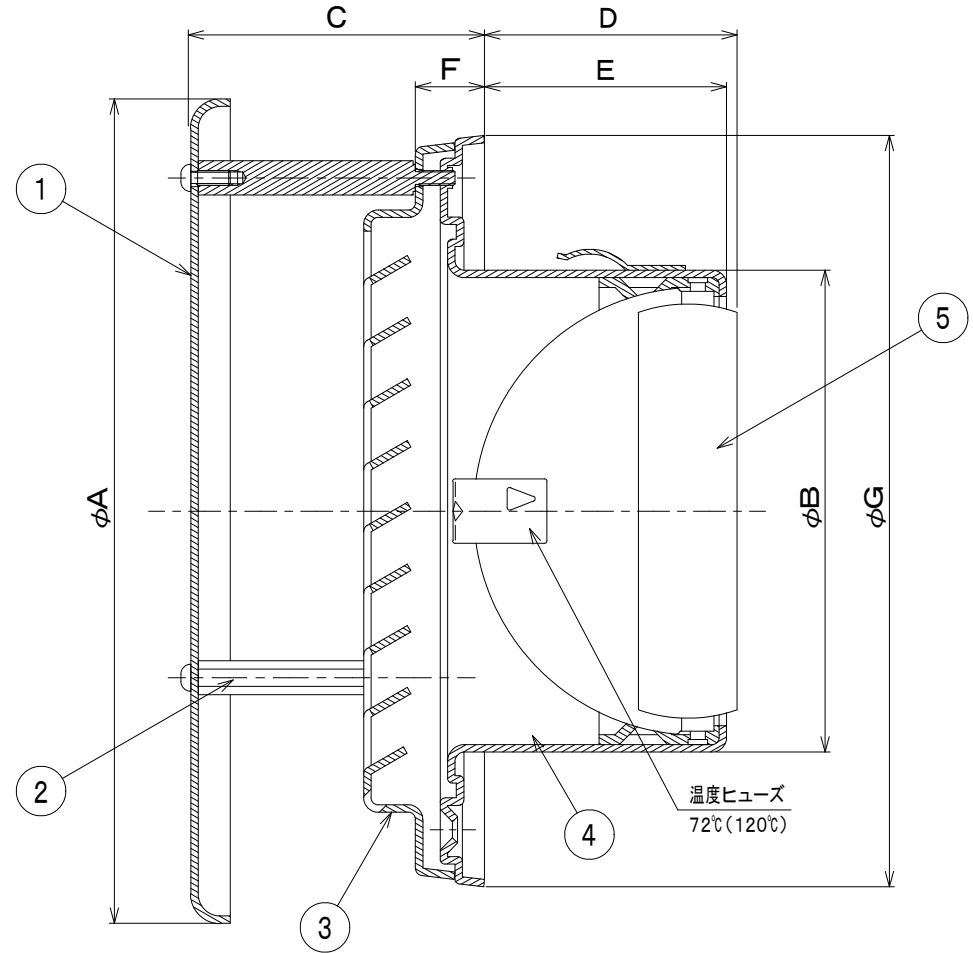
断面 A-A
