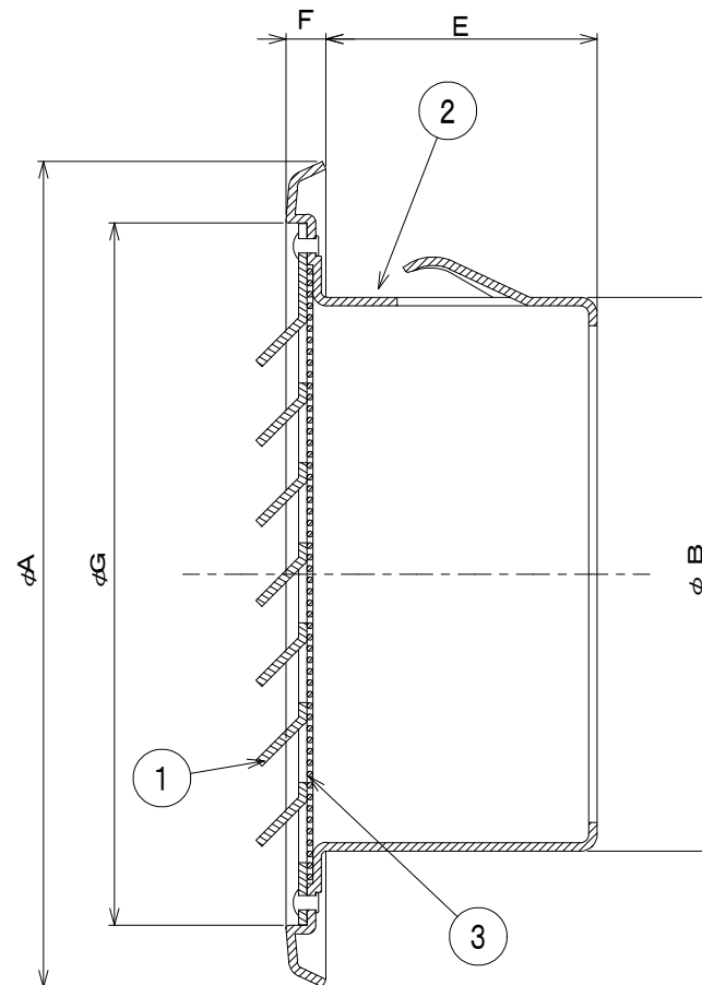
A-A
