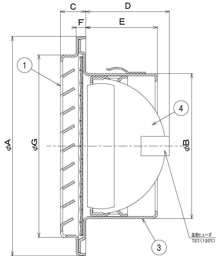
断面A-A
