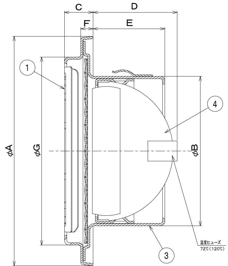
断面A-A
