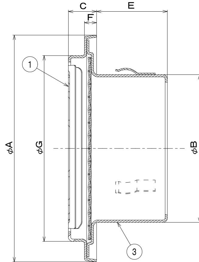
断面A-A
