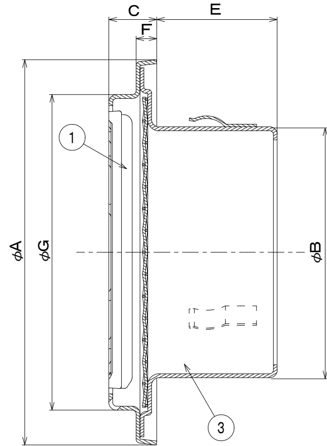
断面A-A
