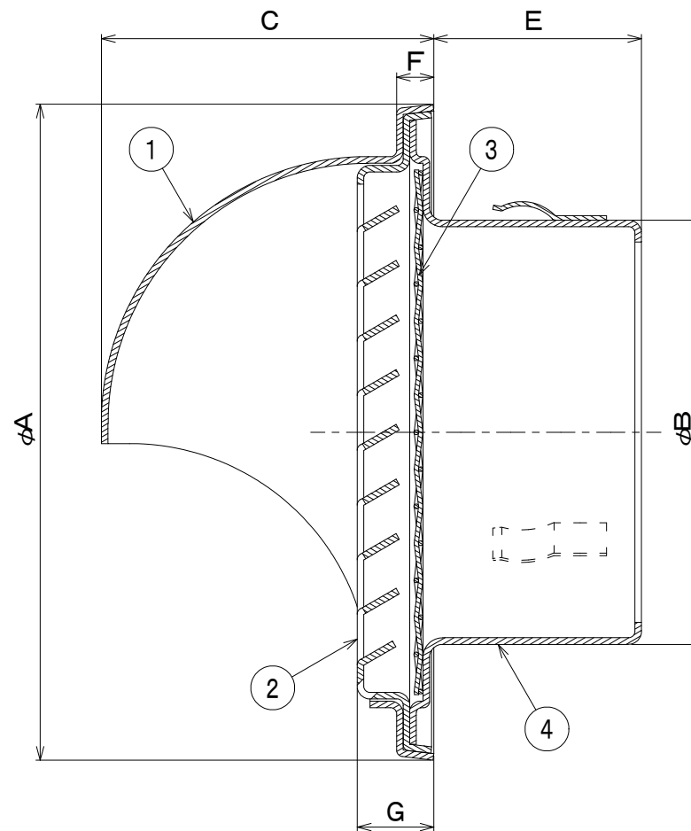
断面A-A
