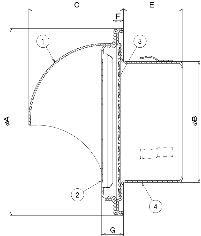
断面A-A
