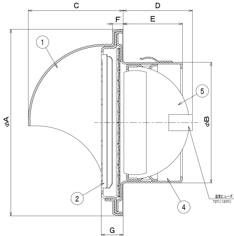
断面A-A
