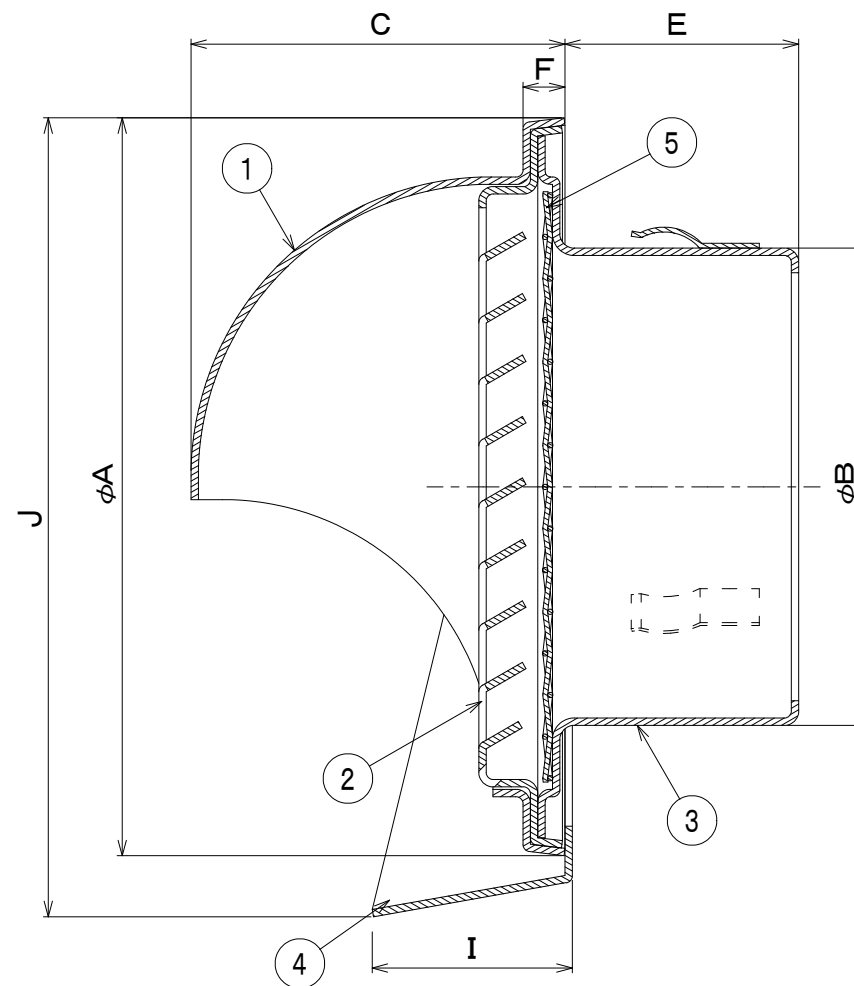
断面A-A
