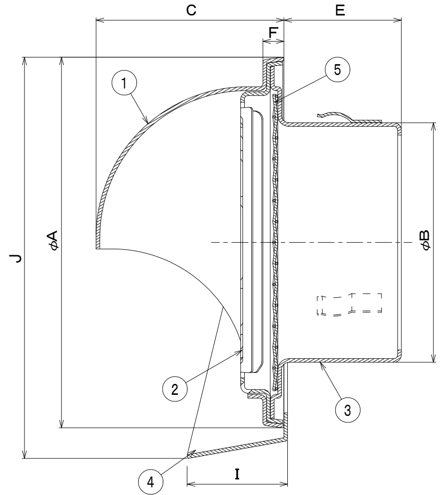
断面A-A
