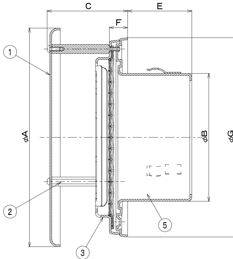
断面 A-A
