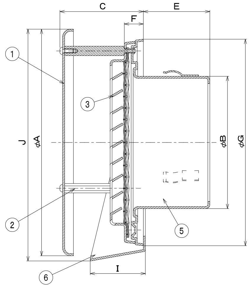
断面 A-A
