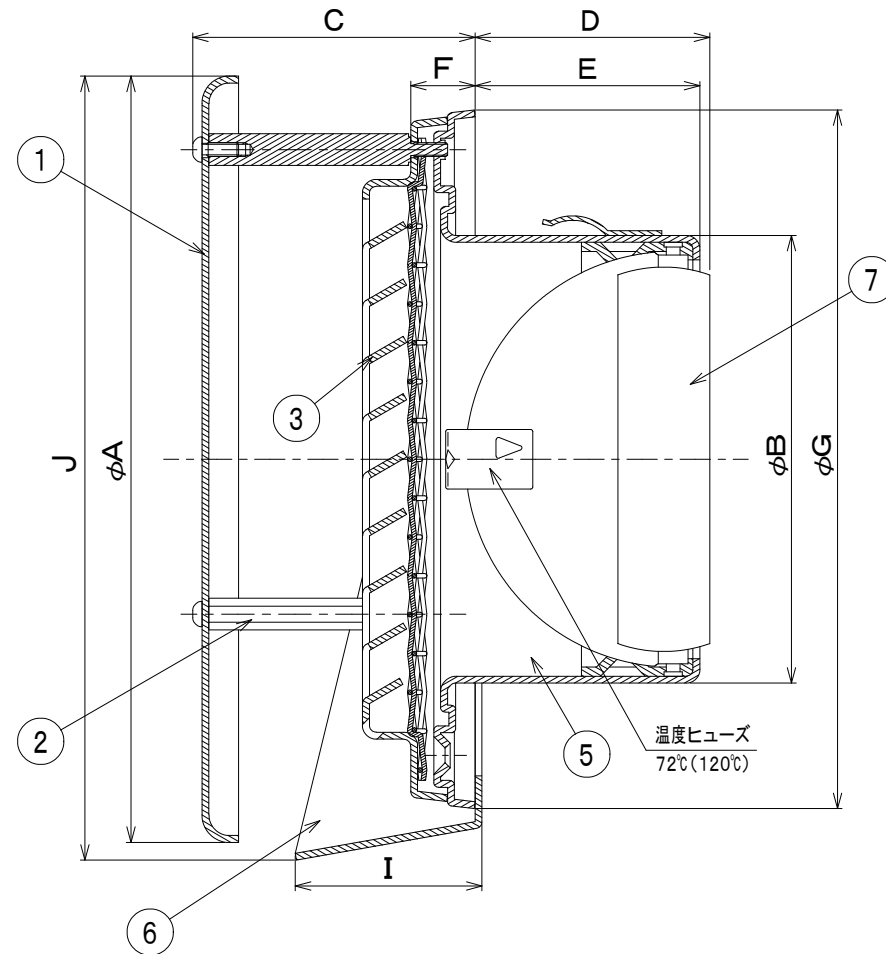
断面 A-A
