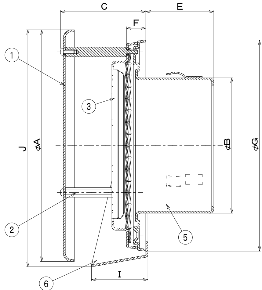
断面 A-A
