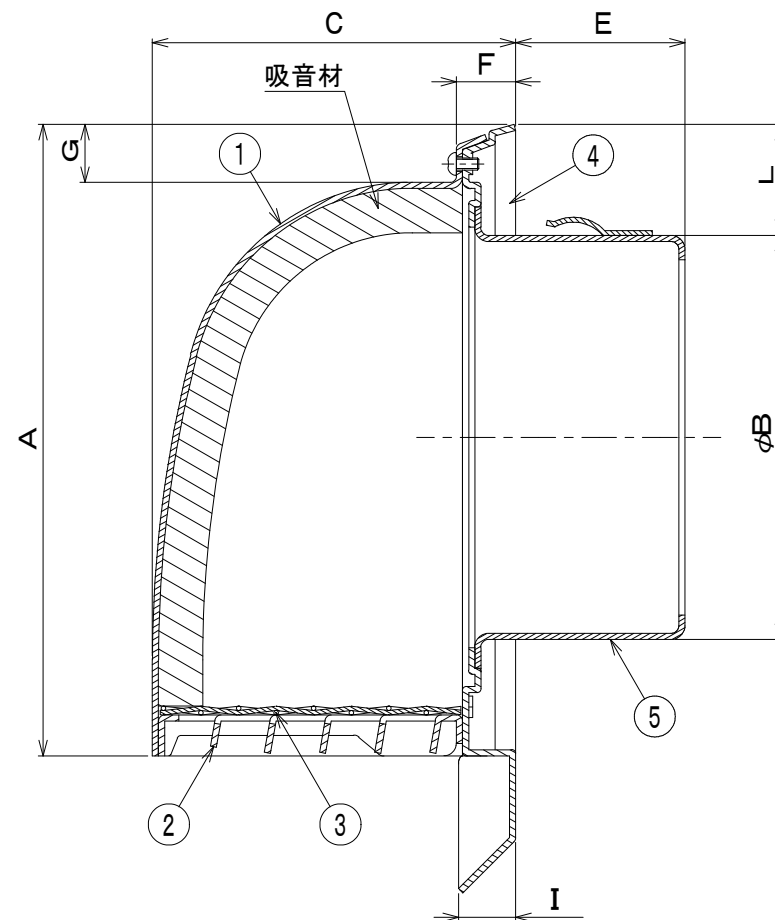
断面 A-A
