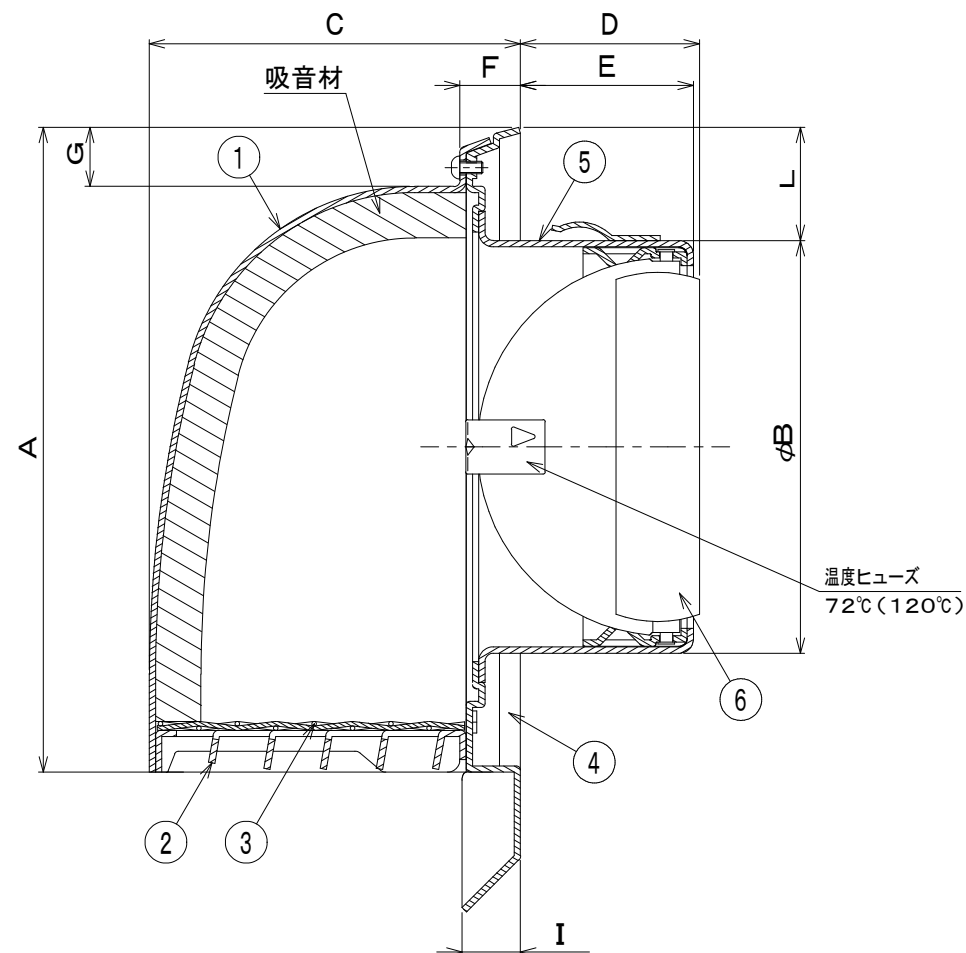
断面 A-A
