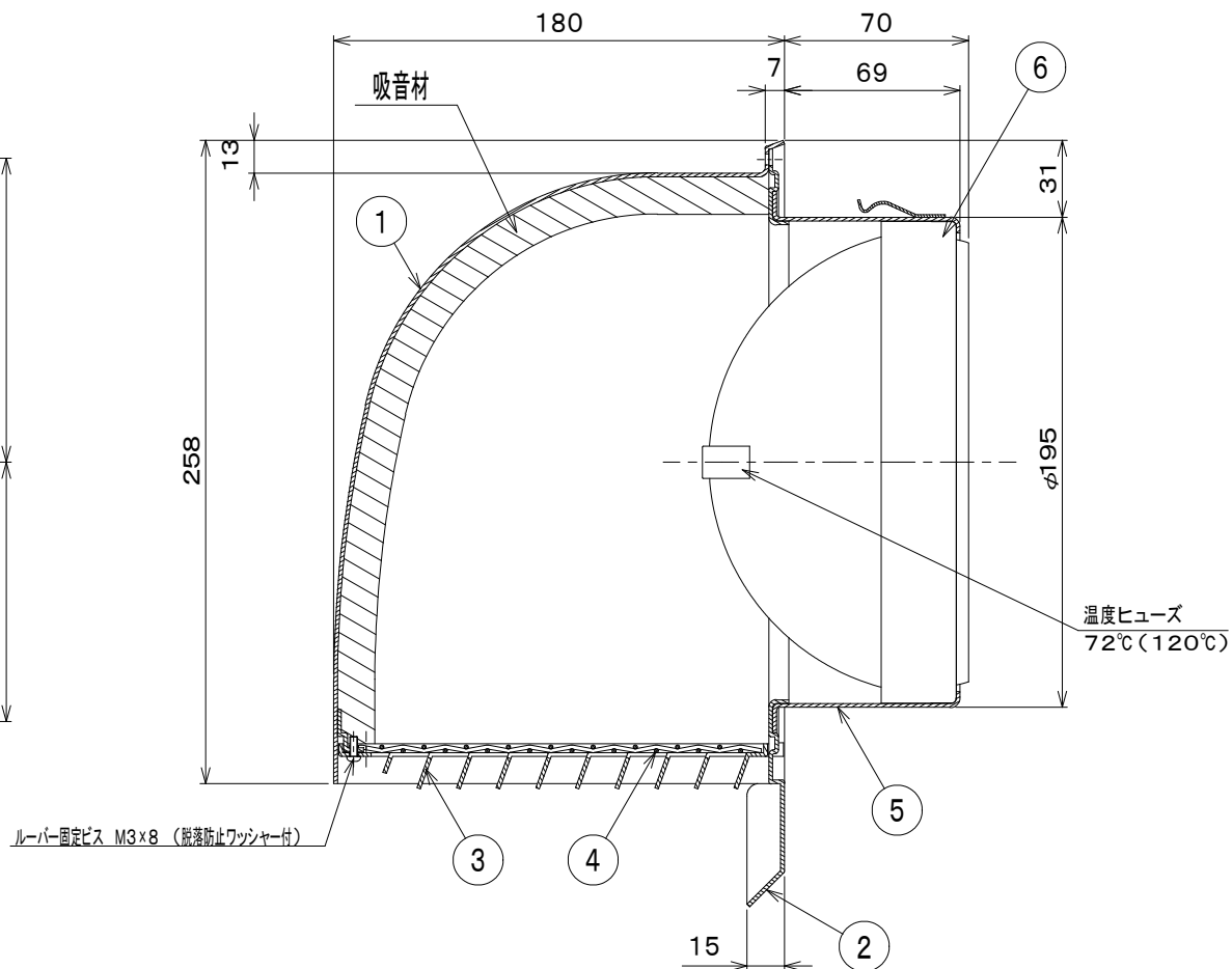
断面A-A
