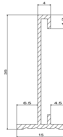
内枠、外枠 断面詳細図
