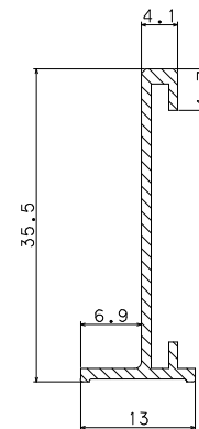
外枠 断面詳細図
