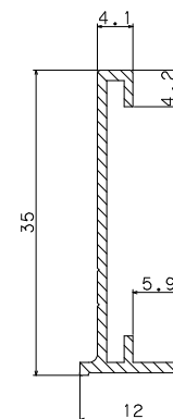
内枠 断面詳細図
