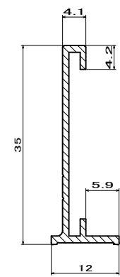
内枠 断面詳細図
