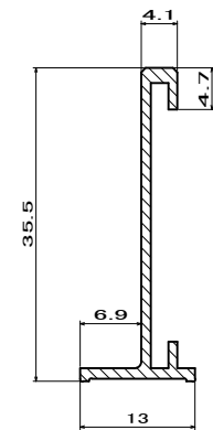
外枠 断面詳細図
