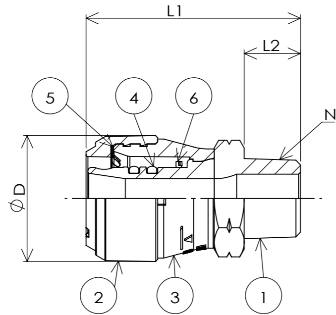
断面図 A-A
