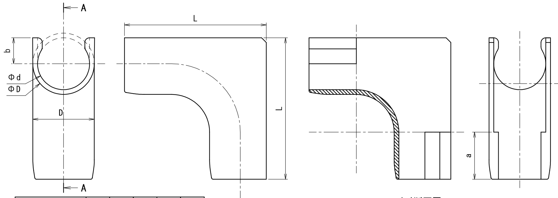
A-A断面図
