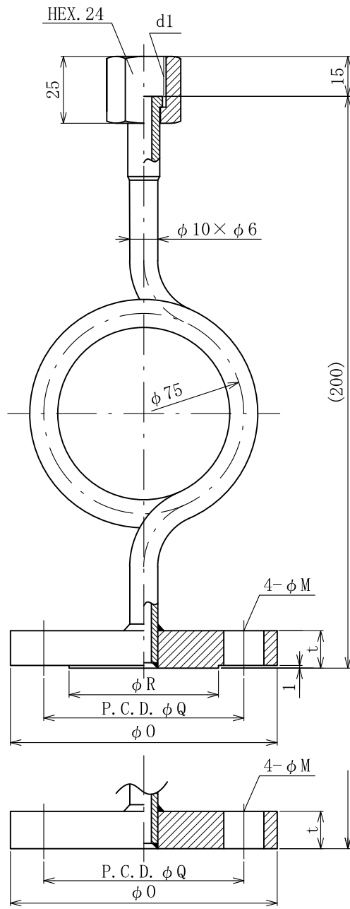
取合フランジ FLANGE CONNECTION 【JIS B2220-2012】
