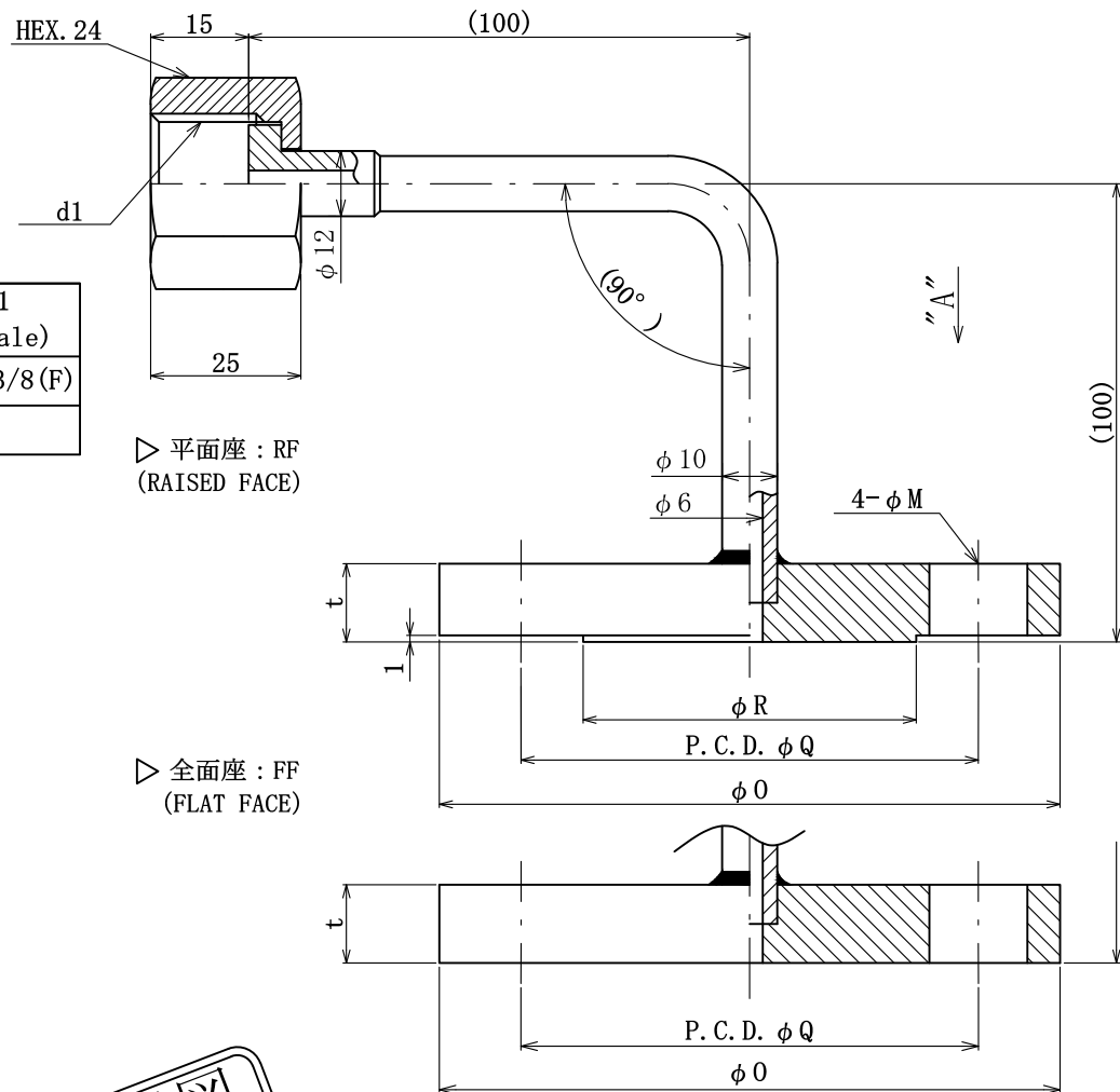
取合フランジ FLANGE CONNECTION 【JIS B2220-2012】
